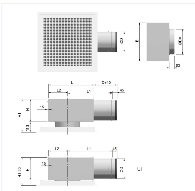
Figur 2, Orion-ATV-T med Luna
