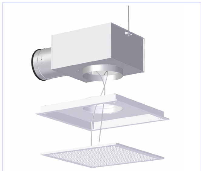
Figur 8, montasje Orion-ATV- T m/luna
