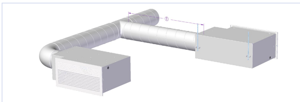
Figur 11, Pegasus-S montasje kanalsystem ① Anbefalt min. 5 x Dia.
