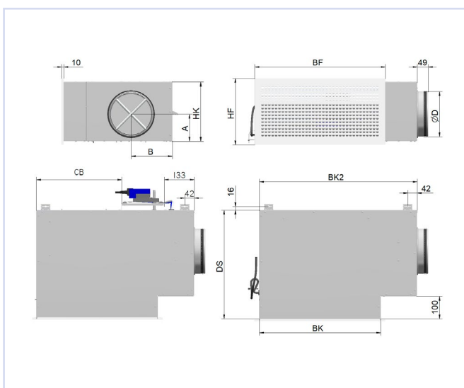
Figur 3, Målskisse Pegasus-S
