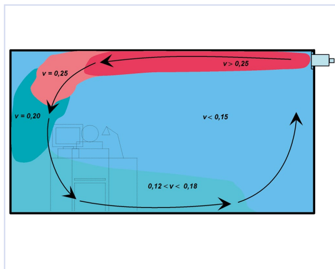
Figur 6, Strømningskisse Pegasus
